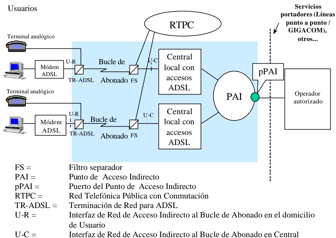
Figura 1: Arquitectura de Red para el Acceso Indirecto al Bucle de Abonado
